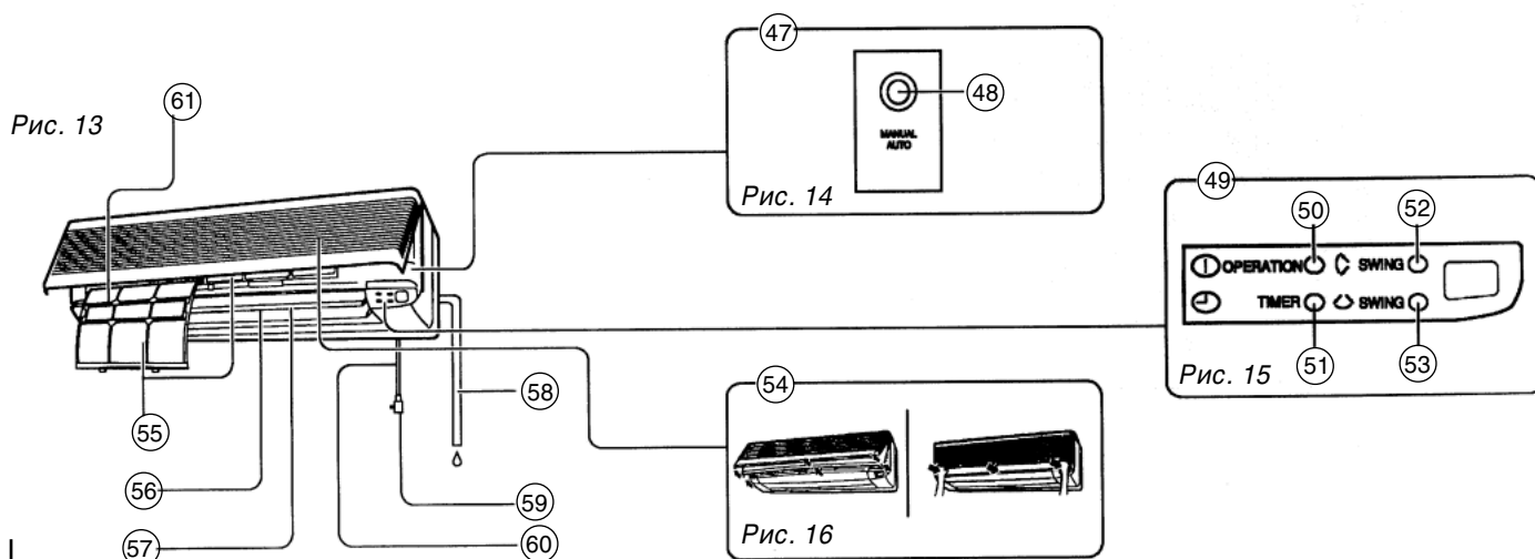
Рис. 13 Внутренний блок
