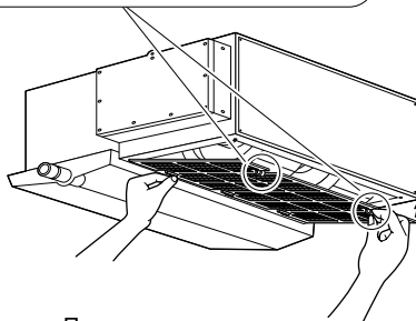
При всасывании снизу.
