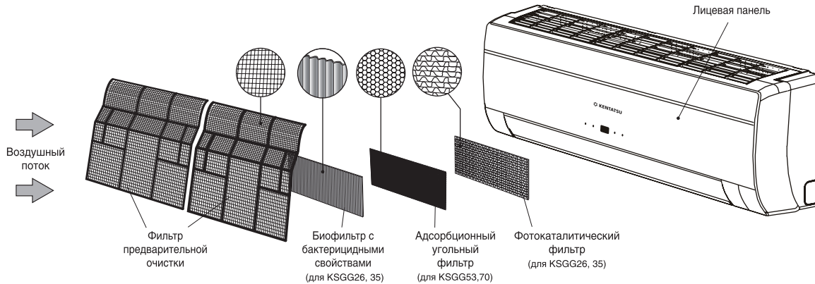
Схема 4-ступенчатой очистки воздуха кондиционером
